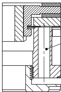
SEZIONE B-B
